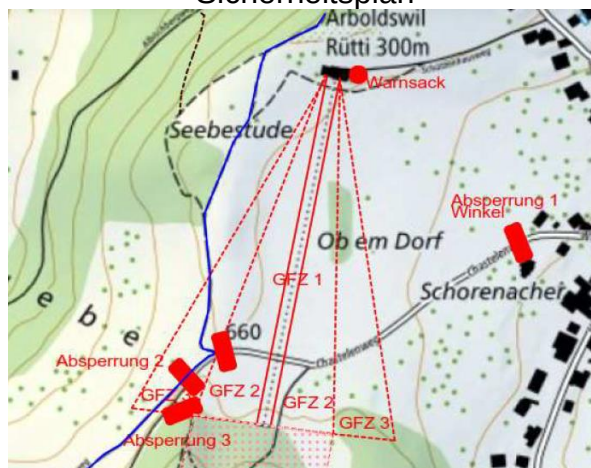
Sicherheitsplan
